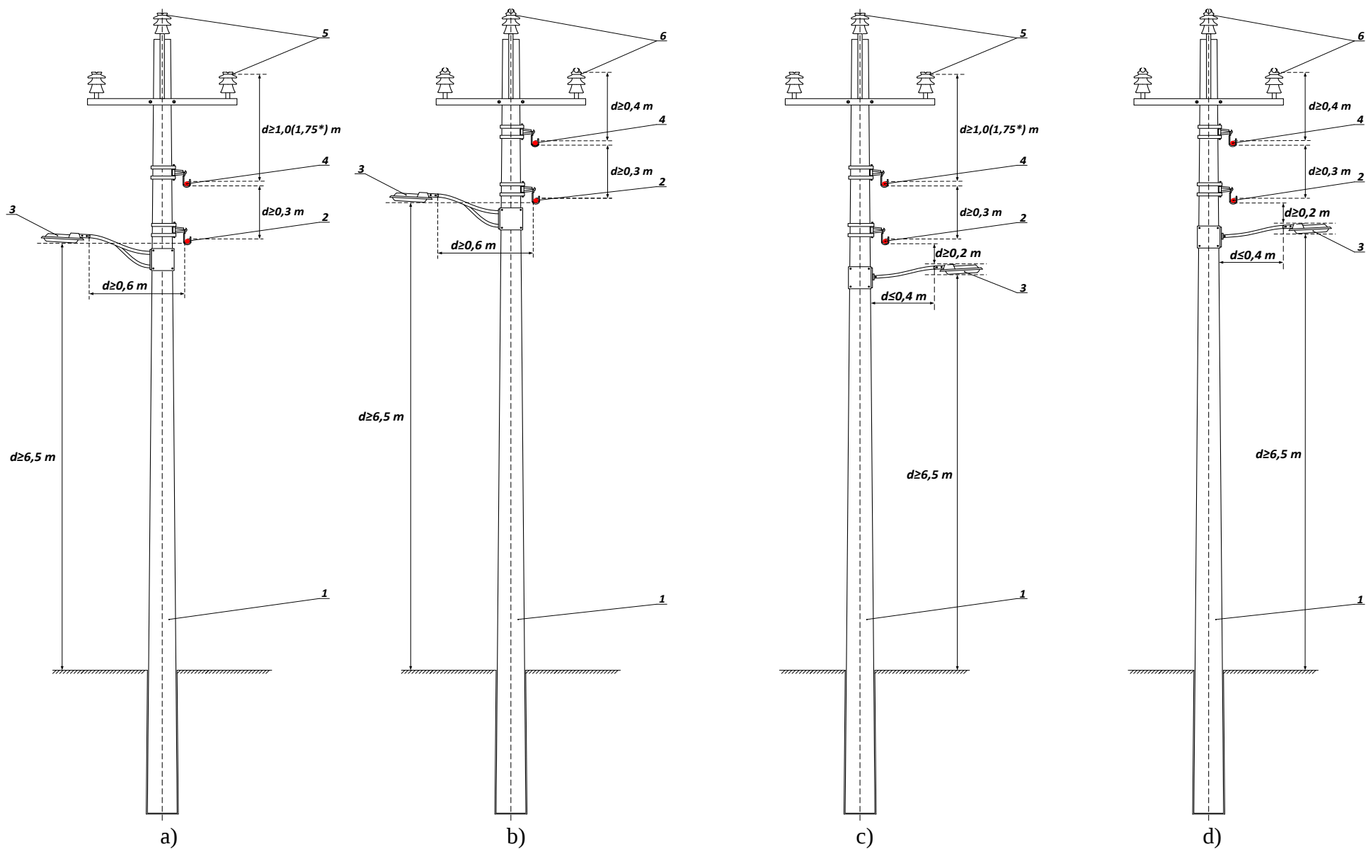
Figura 9. Distanța minimă admisibilă dintre liniile electrice aeriene cu tensiunea (6)10 kV la suspendarea în comun cu LEAI cu tensiunea mai mică de 1000 V cu conductor portant izolat (* - cu conductor portant neizolat) și LEAIP cu amenajarea corpurilor de iluminat în plan orizontal cu LEAIP din diferite părți ale stâlpului sau mai jos de conductoarele LEAIP:
