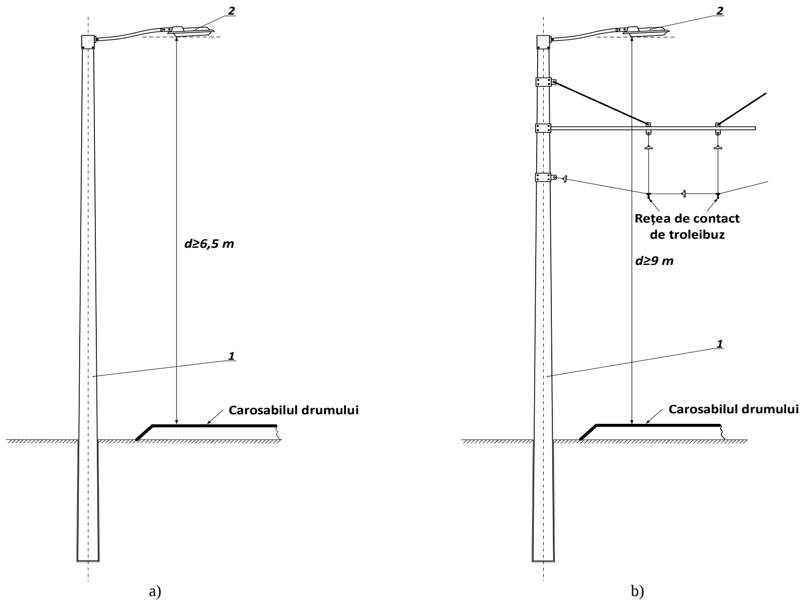
Figura 2. Distanța minimă admisibilă de amenajare a corpurilor de iluminat de la partea carosabilă a drumului și piețelor. Montarea corpurilor de iluminat pe stâlpi ai rețelei de iluminat (a) și montarea corpurilor de iluminat pe stâlpi ai rețelei electrice de contact a transportului electric (b):
