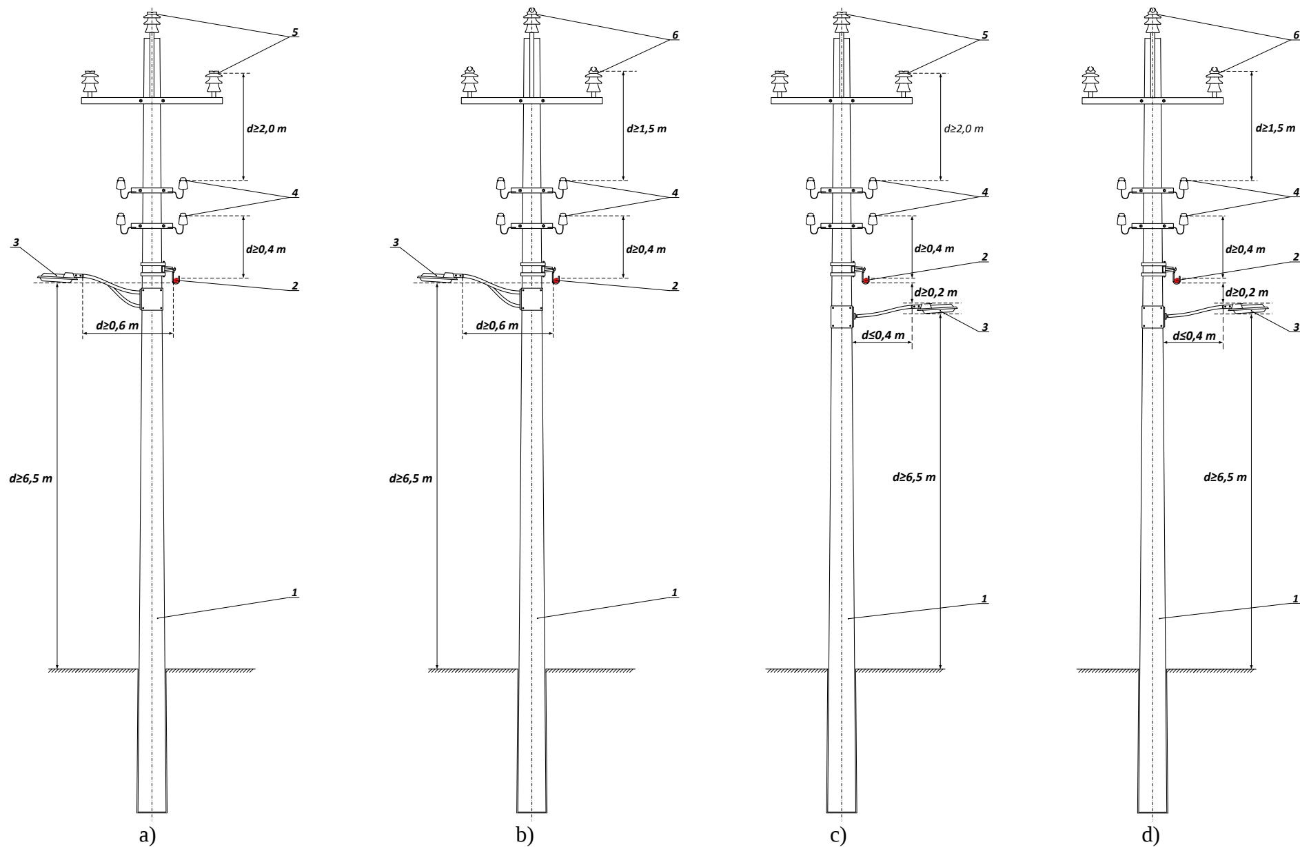
Figura 8. Distanța minimă admisibilă dintre liniile electrice aeriene cu tensiunea (6)10 kV la suspendarea în comun cu LEA cu tensiunea mai mică de 1000 V și LEAIP cu amenajarea corpurilor de iluminat în plan orizontal cu LEAIP din diferite părți ale stâlpului sau mai jos de conductoarele LEAIP: 1 – stâlp, 2 – LEAIP, 3 – corp de iluminat, 4 – LEA cu tensiunea mai mică de 1000 V, 5 – LEA (6)10 kV, 6 – LEAP (6)10 kV
