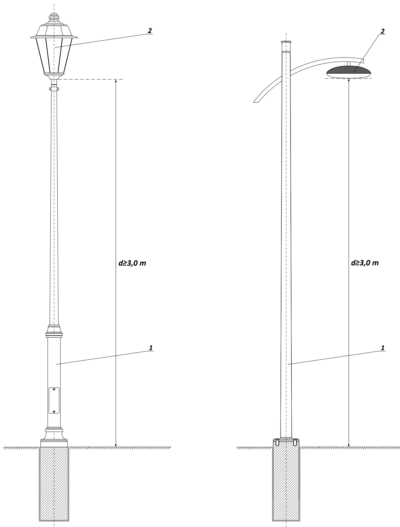
Figura 3. Distanța minimă admisibilă de amenajare a corpurilor de iluminat de la nivelul suprafeței drumurilor pietonale și aleilor: 1 – stâlp, 2 – corp de iluminat
