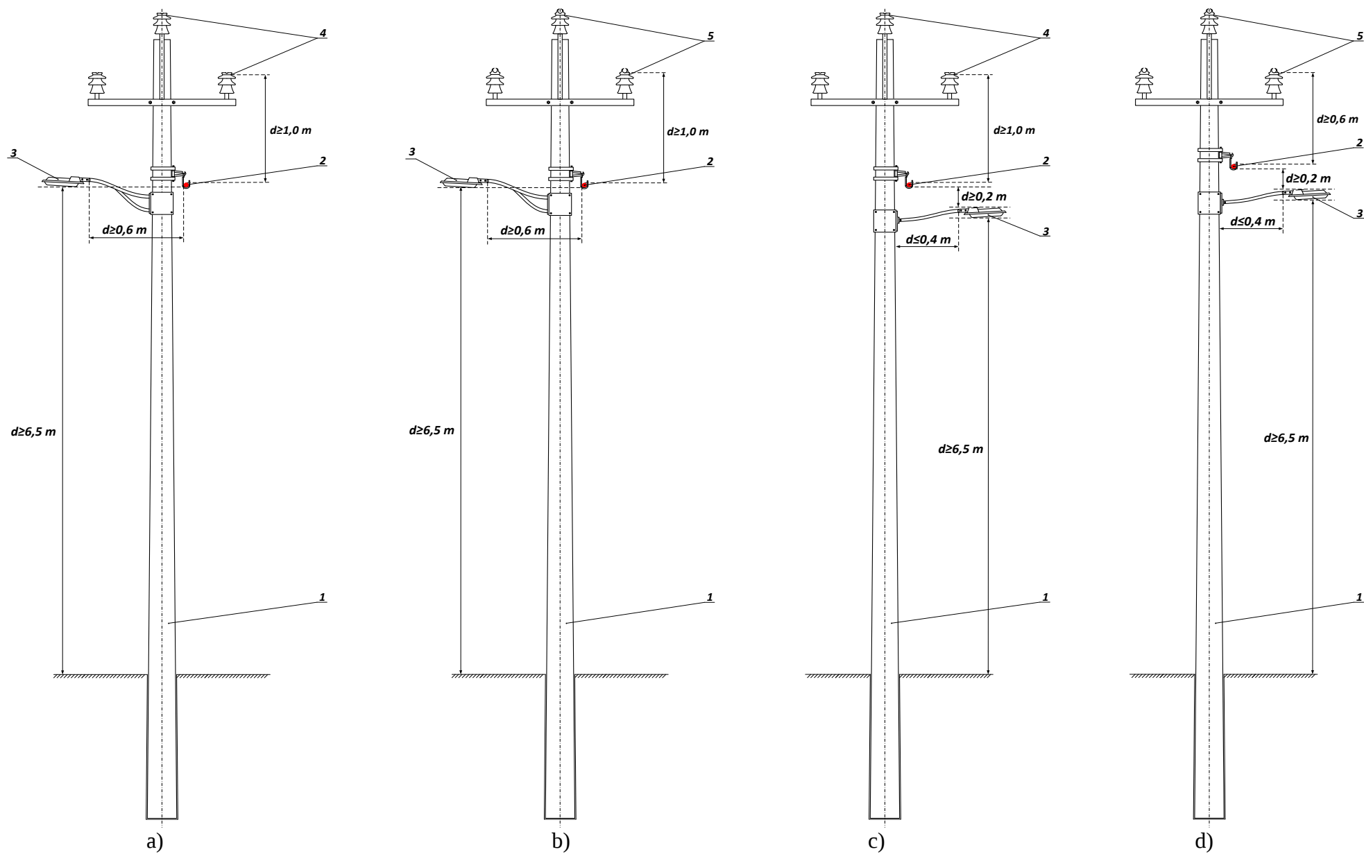
Figura 7. Distanța minimă admisibilă dintre liniile electrice aeriene cu tensiunea (6)10 kV și LEAIP sau LEADIP cu amenajarea corpurilor de iluminat în plan orizontal cu LEAIP din diferite părți ale stâlpului sau mai jos de conductoarele LEAIP: 1 – stâlp, 2 – LEAIP sau LEADIP, 3 – corp de iluminat, 4 – LEA (6)10 kV, 5 – LEAP (6)10 kV
