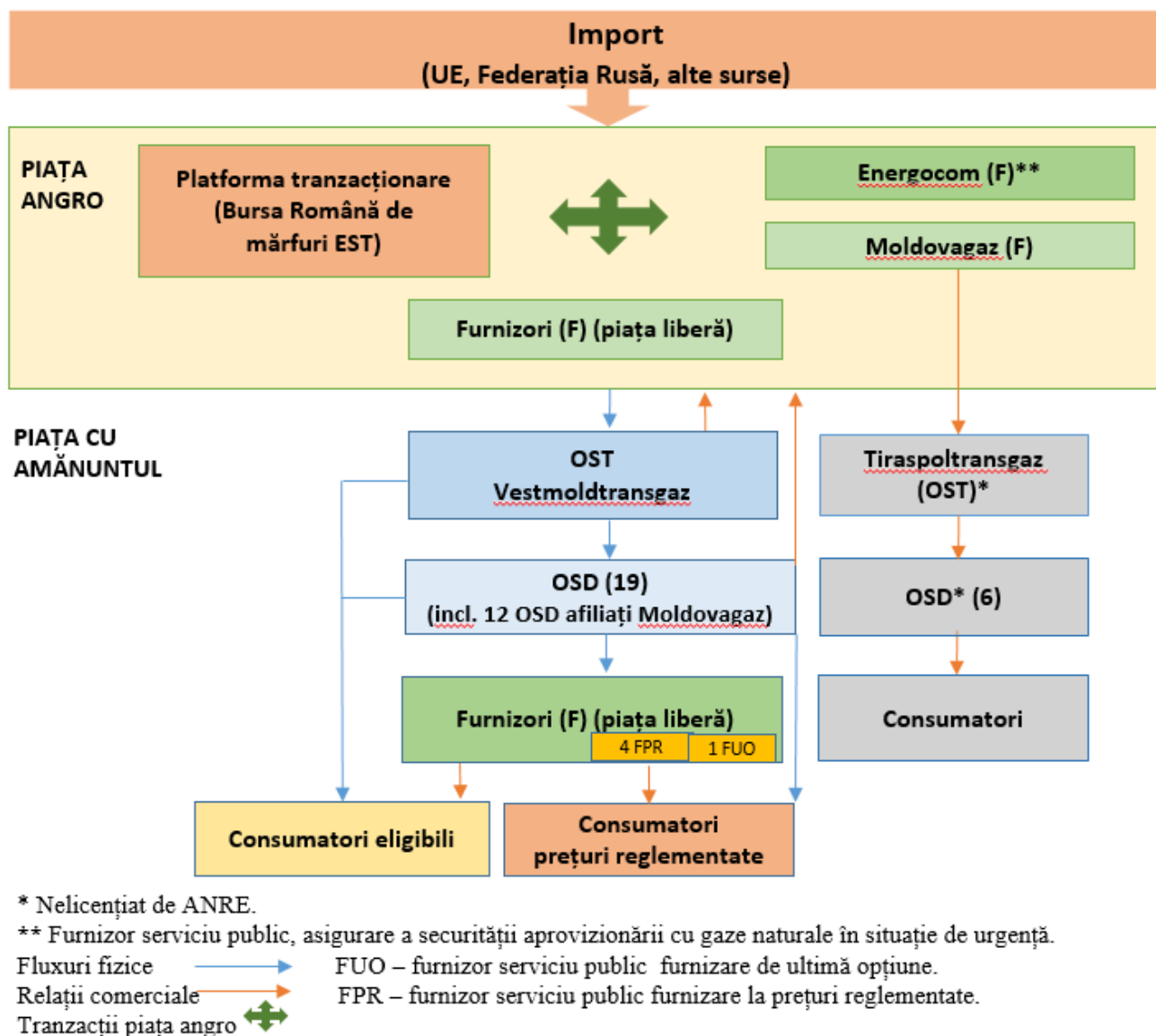
Figura 1. Schema pieței gazelor naturale din Republica Moldova, 2023.
